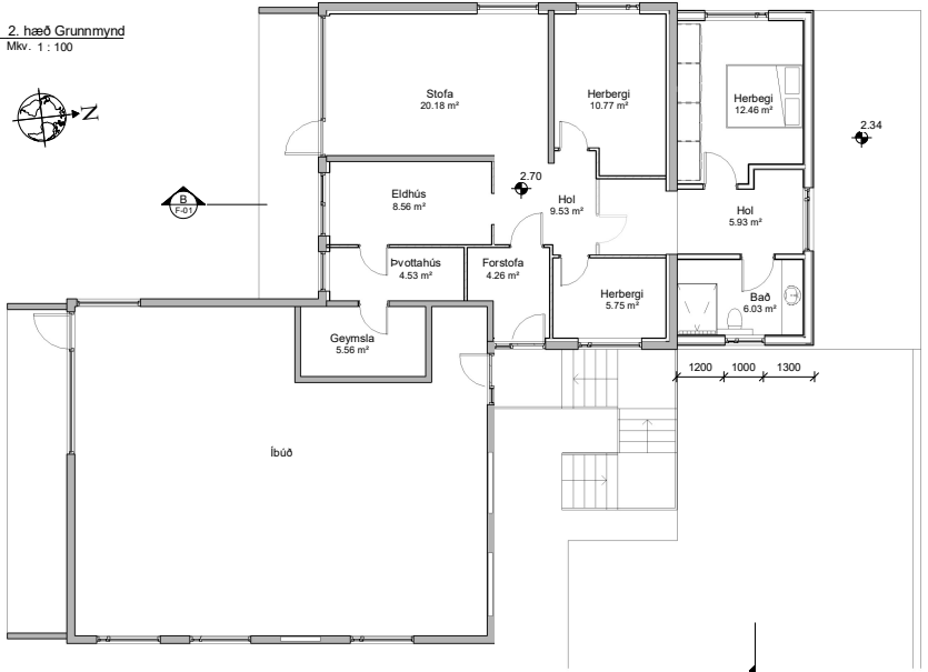
4. hæð Grunnmynd Mkv. 1 : 100
