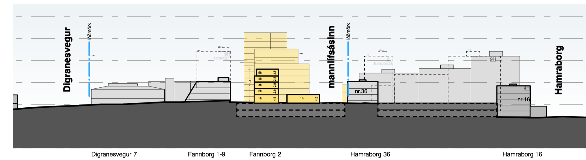
SKILMÁLASNEIÐING F-F
