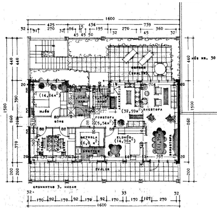
GRUNNMYND 3.HÆÐAR FYRIR BREYTINGU
