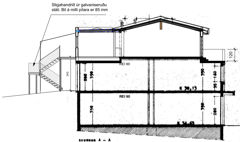
SNEIÐING FYRIR BREYTINGU
