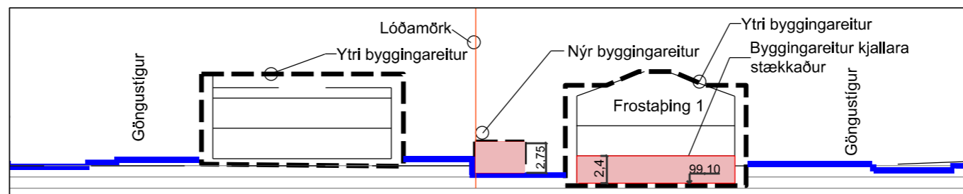
Tillaga að breyttu deiliskipulagi: Sneiðmynd A-A í mkv. 1:500 Kópavogur 3. maí 2021
