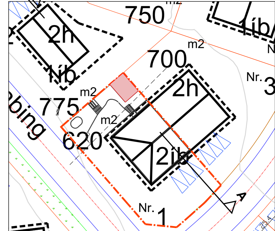
Tillaga að breyttu deiliskipulagi: Afstöðumynd Frostapings 1, í mkv. 1:500
