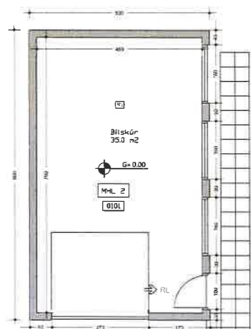
Grunnmynd Bílskúr
