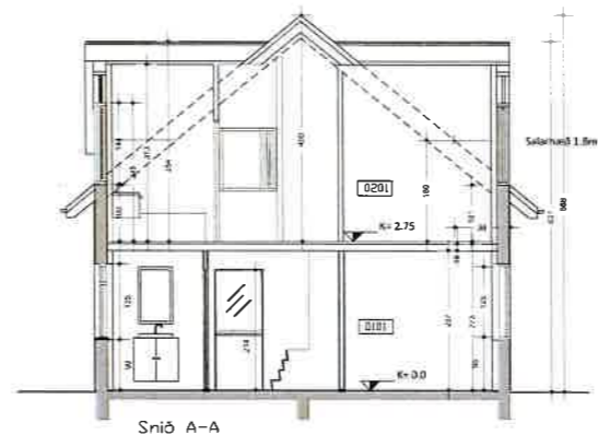
Snið A-A
