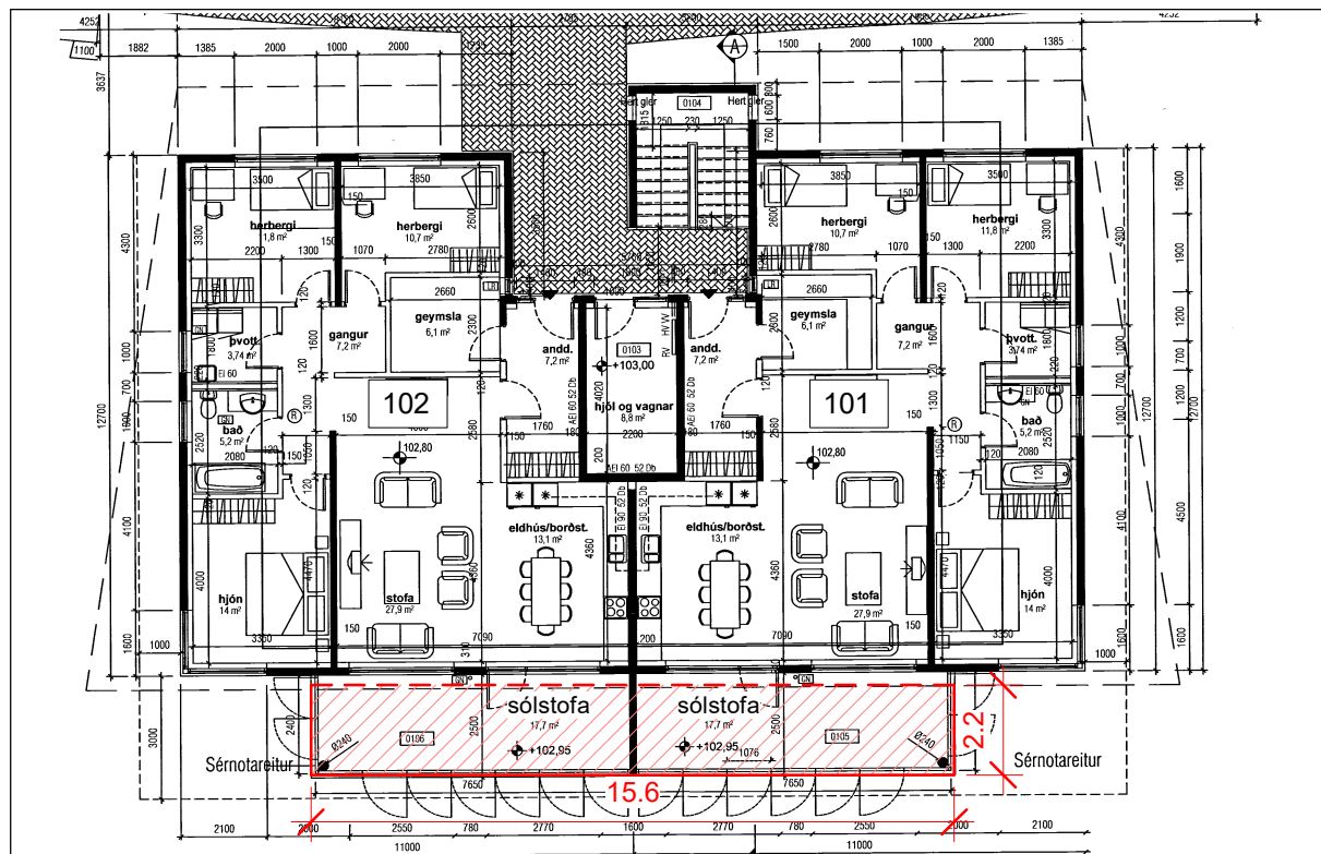
Skýringarmynd. Grunnmynd Baugakór 10 - stækkun byggingarreits við íbúð 101 undirlag: 1:200 gildandi aðaluppdr. (samþ. 05.11.2020)
